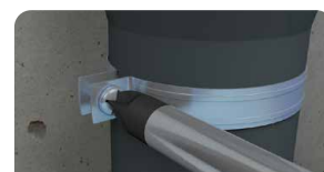
6. Aperte o parafuso da abraçadeira com o binário recomendado
