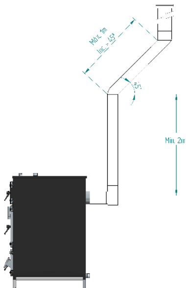
Figura 13 - Exemplo de instalação típica
