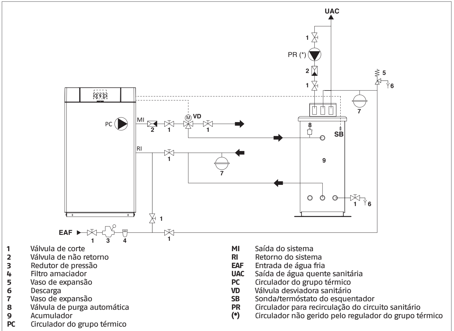
Esquema 2: circuito com grupo térmico ligado diretamente ao sistema de aquecimento e produção de AQS com acumulador e válvula desviadora externa
