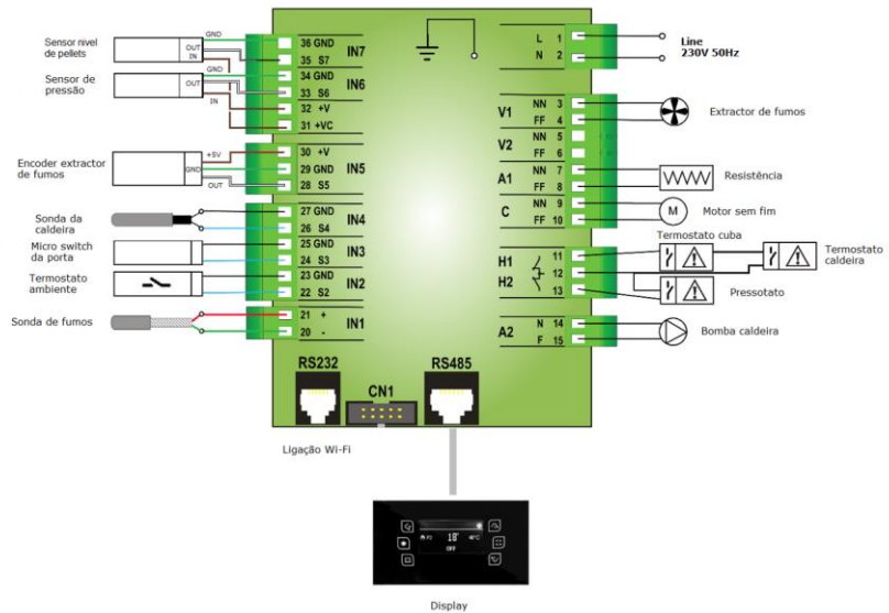
Figura 70 - Esquema elétrico (eletrônica Columbus)
