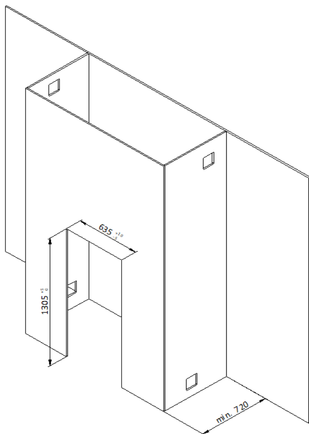
Figura 8 - Medidas saco pladur
