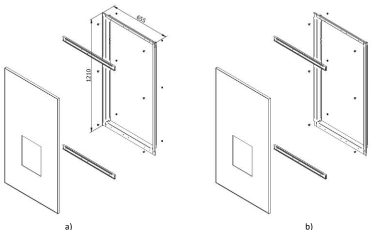
Figura 12 - a) Porta com aro de abertura direita, b) Porta com aro de abertura esquerda
