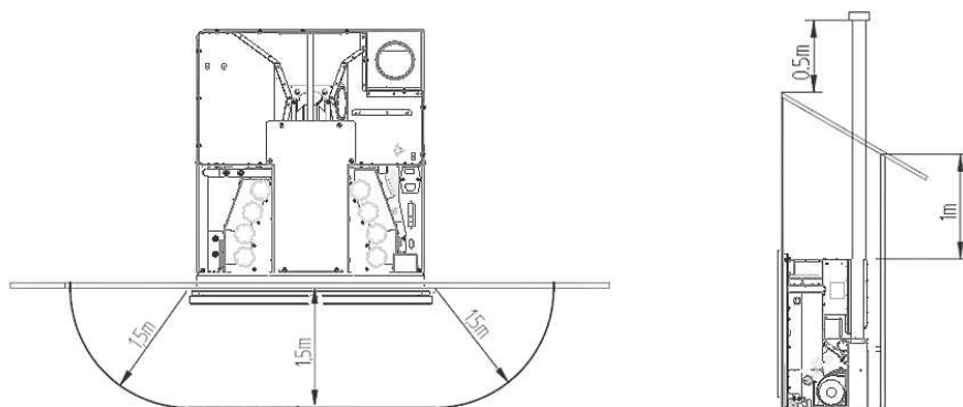
Figura 7 - Distâncias mínimas de todas as superfícies
