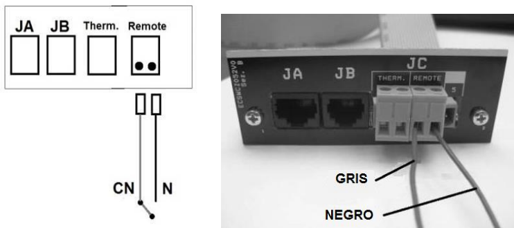
Figura 42 - Ligações do comando externo com fios
