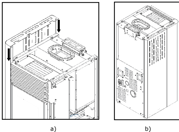
Figura 97 – Fixação laterais das envoltentes
