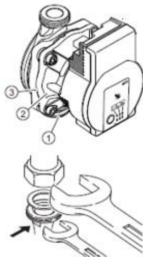
Figura 68 – Instalação da bomba
