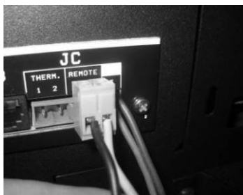
Figura 18 – Ligação do comando remoto sem fios
