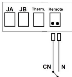
Figura 19 – Ligações do comando externo com fios
