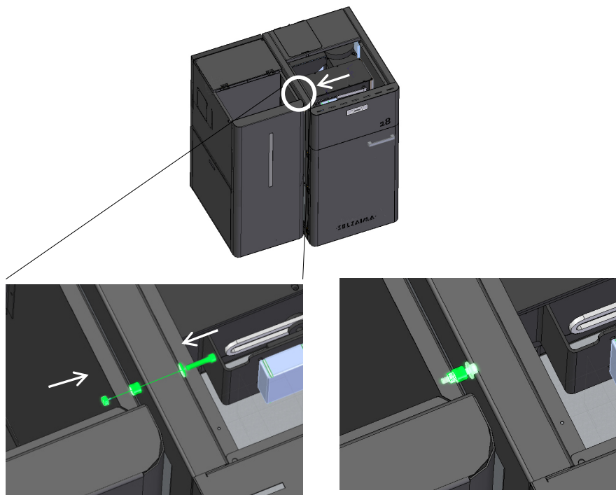
Figura 44 – Fixação lateral do silo à caldeira
