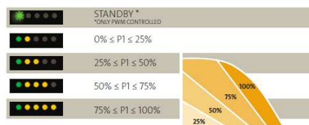
Figura 65 – Níveis de performance da bomba
