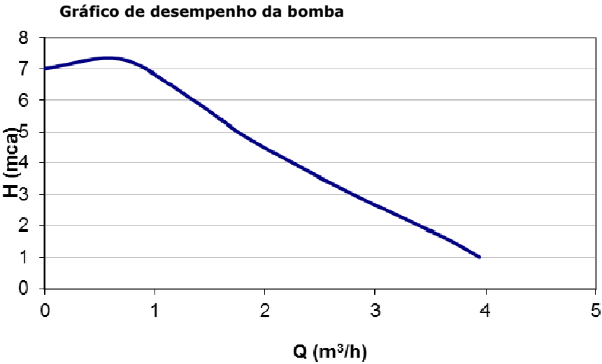
Figura 63 – Gráfico de desempenho da bomba
