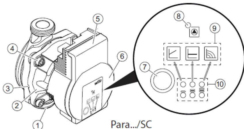
Figura 67 – Bomba Wilo
