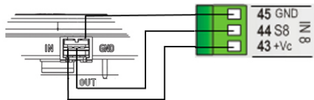
Figura 62 – Ligações do sensor (eletrônica Columbus)
