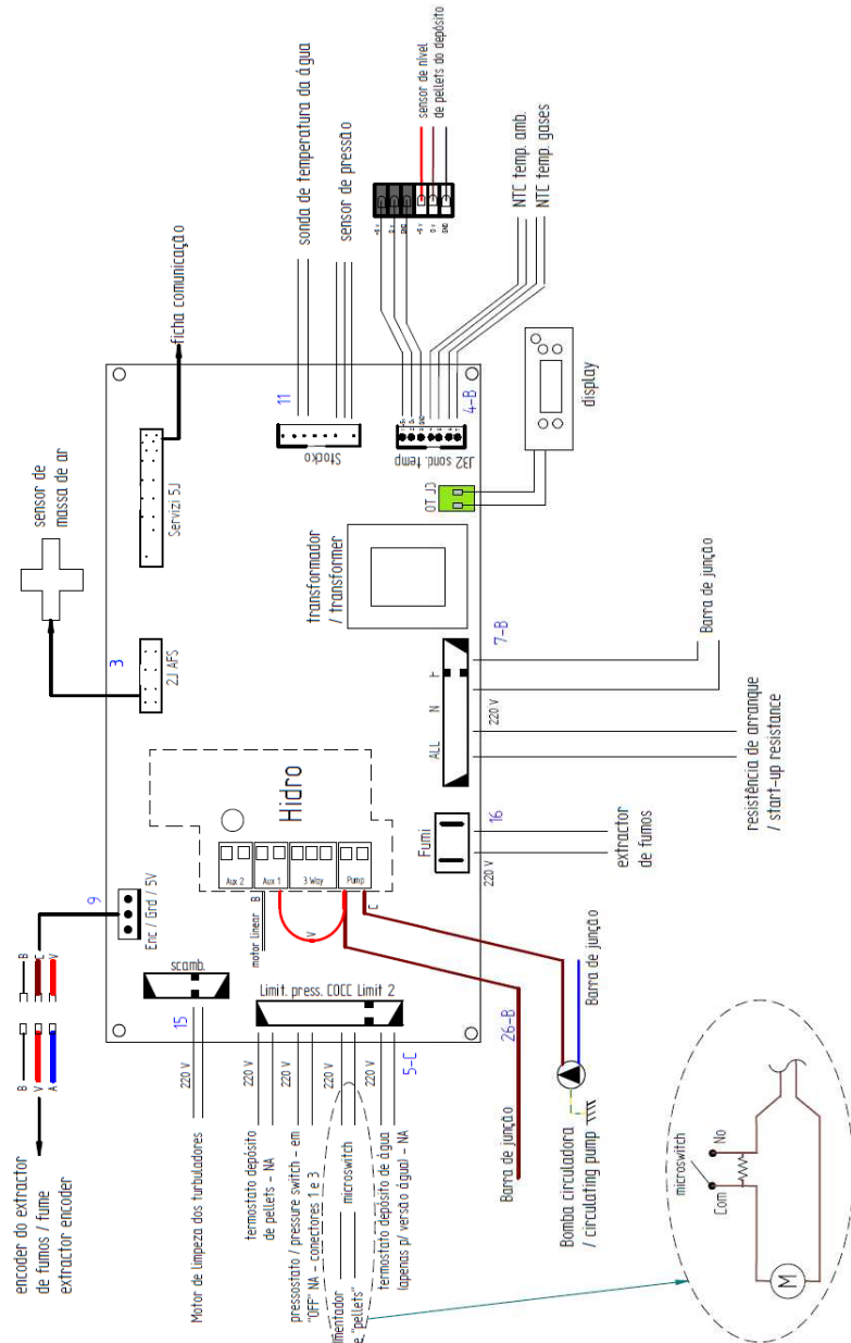
Figura 58 – Esquema elétrico da placa eletrônica
