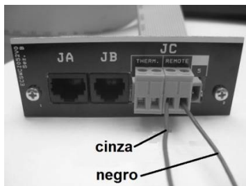
Figura 19 – Ligações do comando externo com fios
